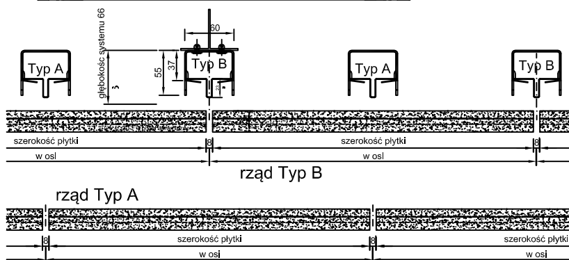
montaż Typ A
