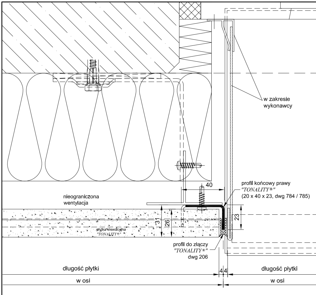
DETAL TYPOWY "7.4" (Rys. ANo. BAS 200-13)
