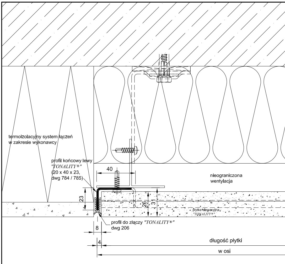
DETAL TYPOWY 10
